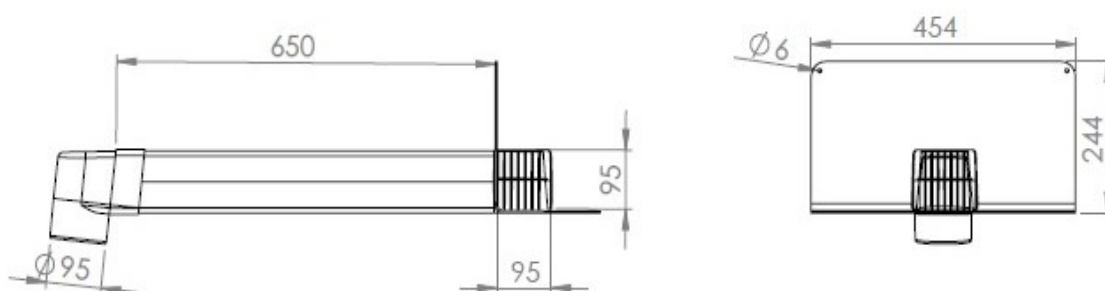
Рис. 1. Схема воронки VC-PVC
